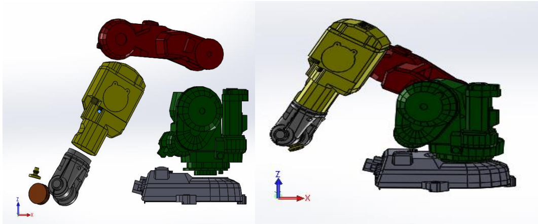
الشكل (1) – أجزاء الروبوت ABB IRB 140 وتجميعها ضمن Solidworks.
