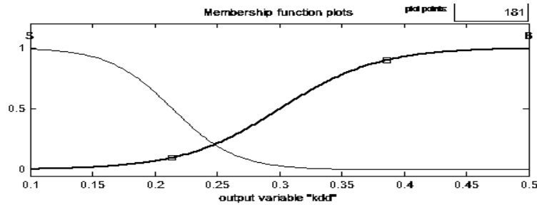
الشكل (8-8) :توابع الانتماء للخروج K_{aa}
