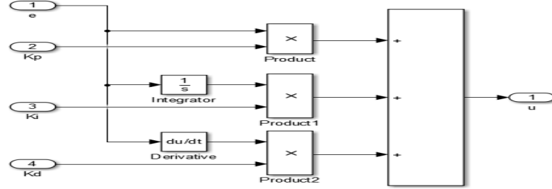
الشكل (5) - نموذج متحكم PID.
