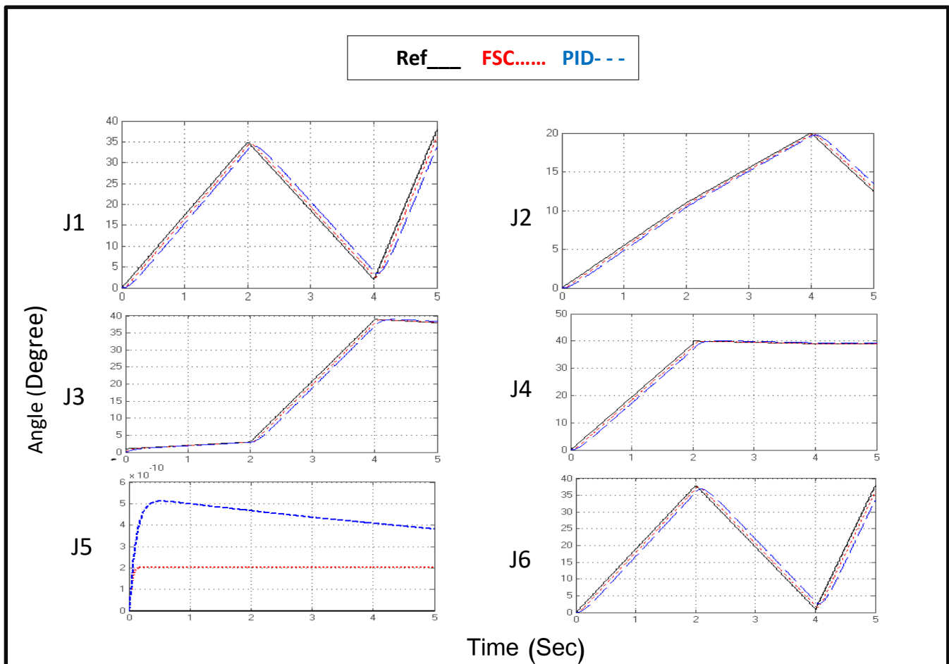
الشكل (12) - الخطأ الثابت عند استخدام PID و FSC مع دخل متغير.
