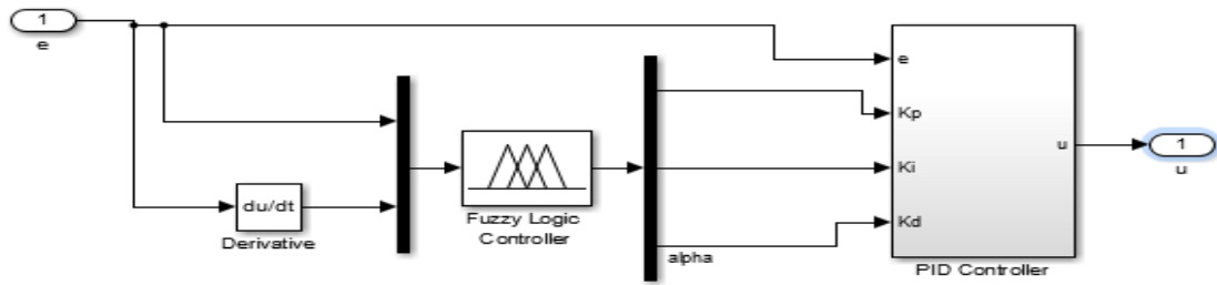
الشكل (6) - المتحكم (FSC) في بيئة Simulink.
