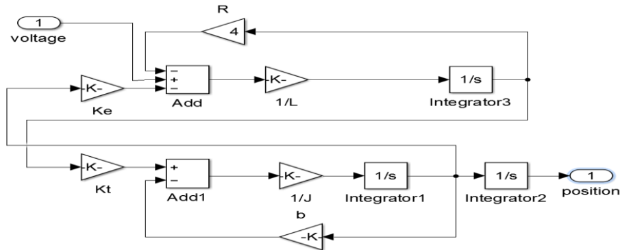
الشكل (3) - نموذج Simulink لدارة محرك DC.
