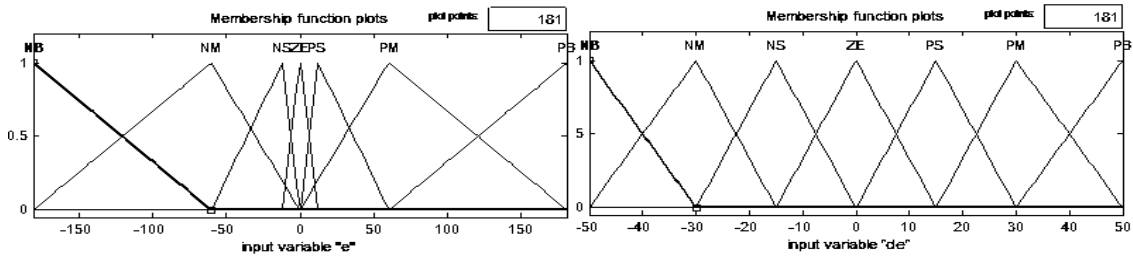
الشكل (7-a) : توابع الانتماء للخطأ (e)
