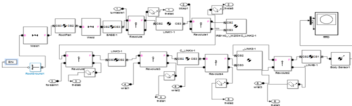
الشكل (2) – نموذج Simulink الناتج عن تنفيذ Simscape Multibody للمناول ABB IRB 140.
