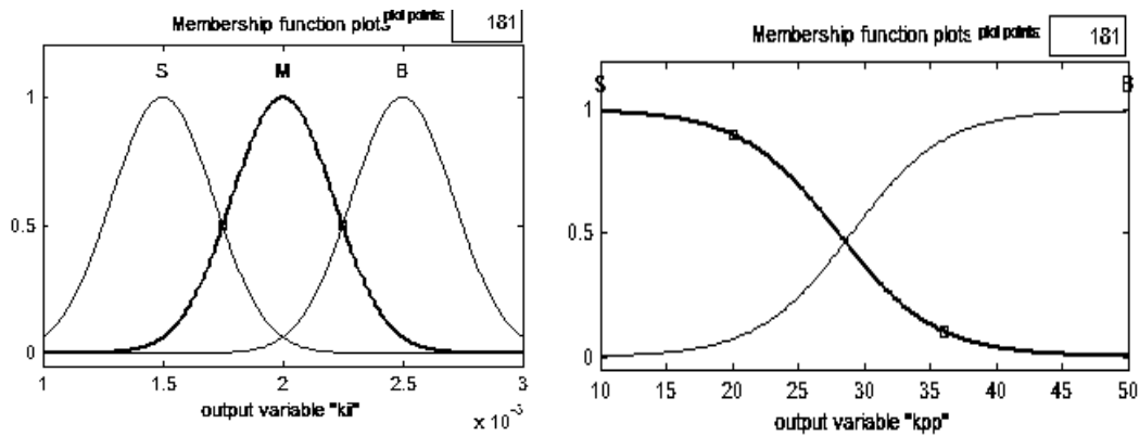
الشكل (8-a) : توابع الانتماء للخرج K_{pp}
