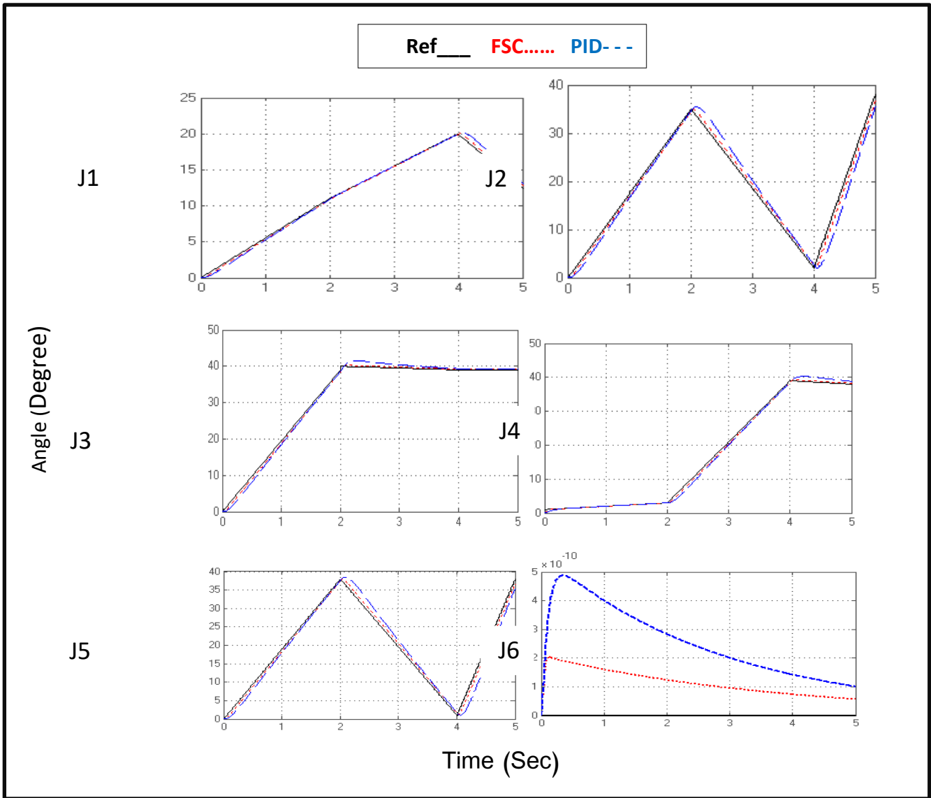
الشكل (13)- الخرج الناتج عن استخدام PID و FSC عند دخل متغير بعد تعديل بارامترات التحكم.
