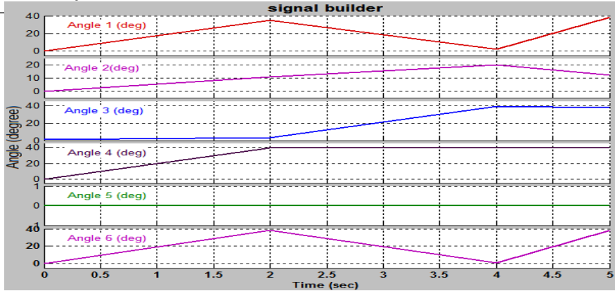
الشكل (11) - إشارة دخل متغيرة على المفاصل الستة.
